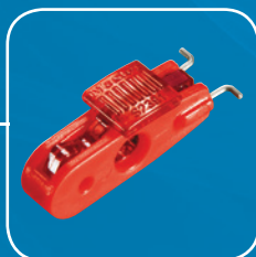
S2391 - Patillas metálicas hacia el exterior : distancia de 11 a 13mm
